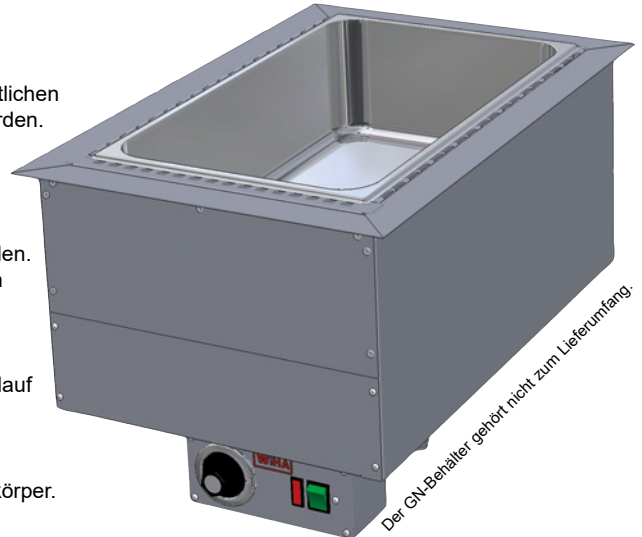
Der Thermostat kann alternativ in eine Thekenblende eingebaut werden (Leitungslänge ca. 45 cm).
