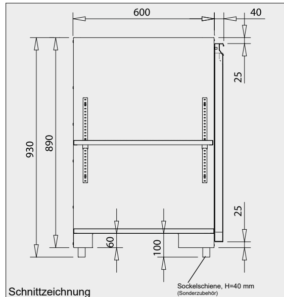
Schnittzeichnung
