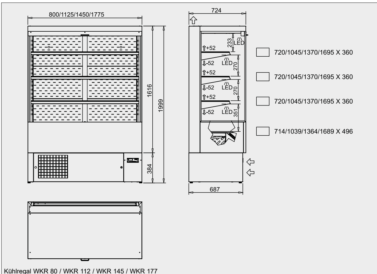
Kühlregal WKR 80 / WKR 112 / WKR 145 / WKR 177
