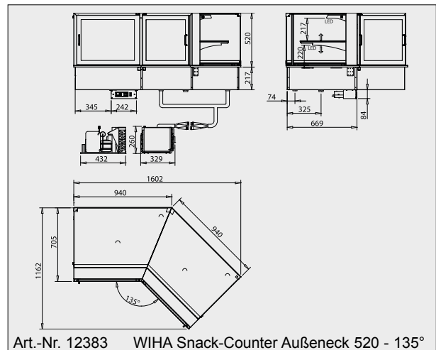
Art.-Nr. 12383 WIHA Snack-Counter Außeneck 520 - 135°
